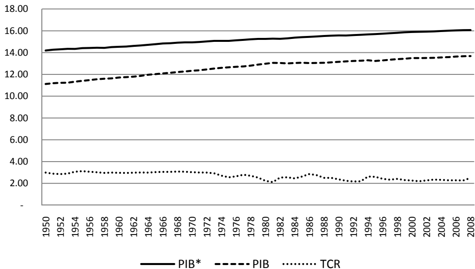
Gráfico 4.2 PIB, PIB* y TCR (Logaritmos)
