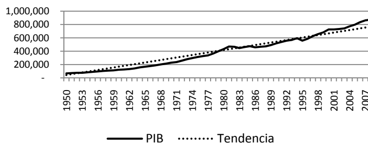
Gráfico 6.1 PIB Y SU TENDENCIA*
