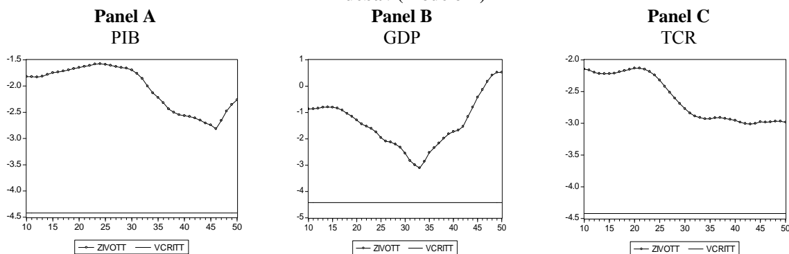
Gráfico 4.5 Prueba t (Modelo B)
