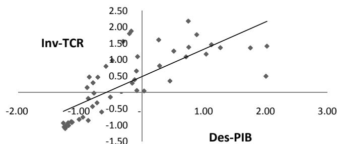
Gráfico 6.4 VALORES ESTANDARIZADOS DE DESVIACIONES DEL PIB DE SU TENDENCIA Y DEL INVERSO TIPO DE CAMBIO REAL (1960-2008)
