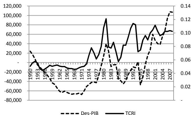
Gráfico 6.2 DESVIACIÓN DEL PIB DE SU TENDENCIA E INVERSO DEL TIPO DE CAMBIO REAL (1950-2008 - Datos anuales)
