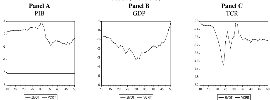
Gráfico 4.6 Prueba t (Modelo C)
