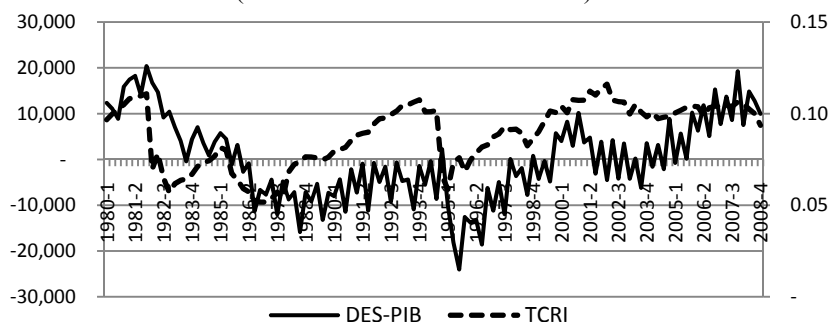
Gráfico 6.3 DESVIACIÓN DEL PIB DE SU TENDENCIA E INVEROS DEL TIPO DE CAMBIO REAL (1980-2008 - Datos Trimestrales)
